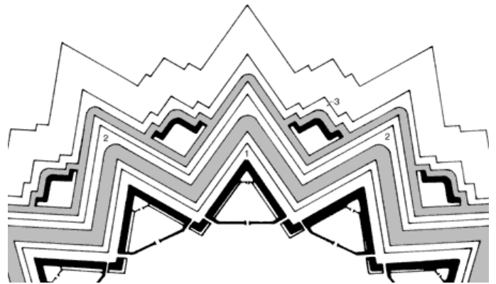
Getenailleerd stelsel : 1. omwalling van tenaille-vormige vestingfronten; 2. doorlopende couvre-face; 3. inspringende wapenplaats
